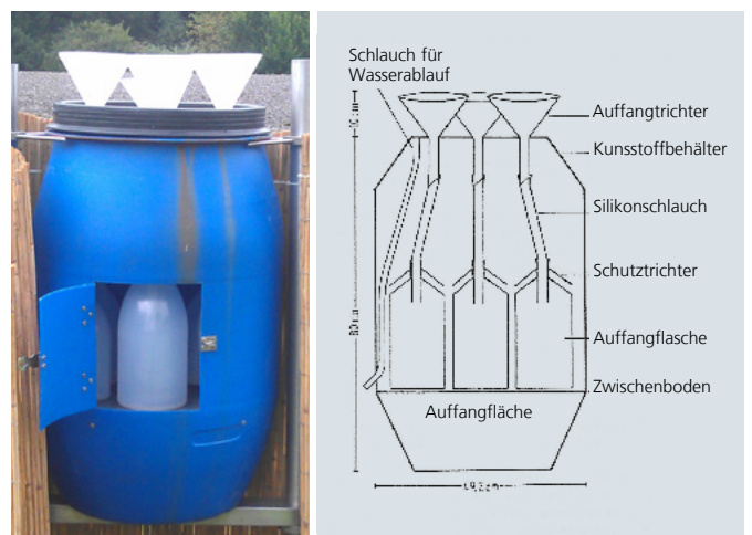
Niederschlagssammler im Freiland.
