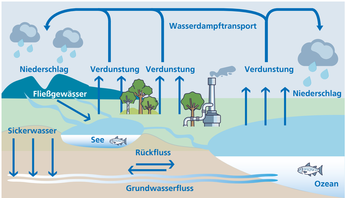
Schematische Skizze des Wasserkreislaufes.
