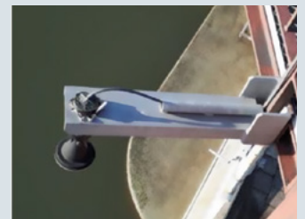
Radarmesssonde des Pegels an der Varel Schluise.
