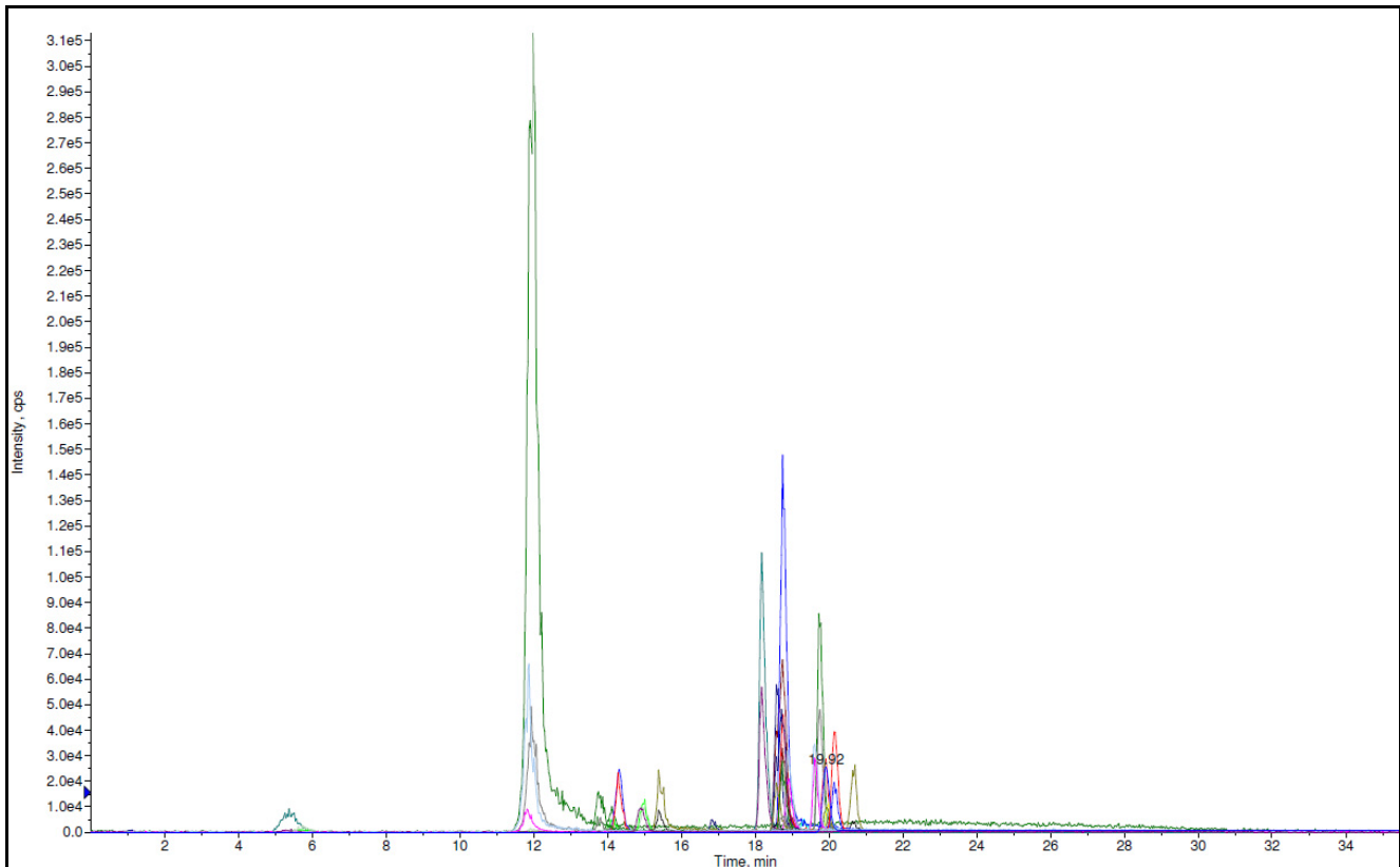
Abbildung 3: Beispiel-Chromatogramm (Standard 500 ng/mL).
